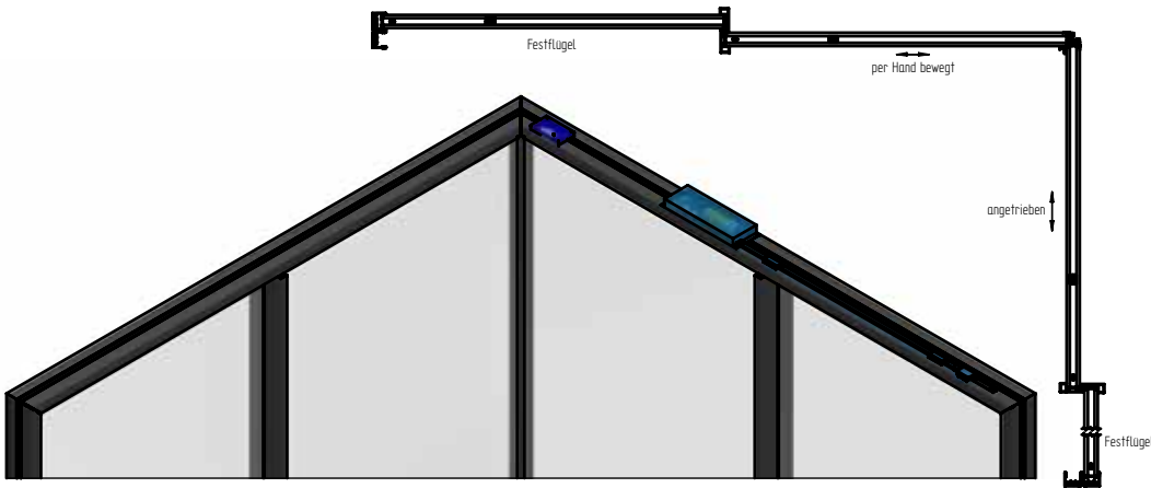
Ecklösung - Teilangetrieben
