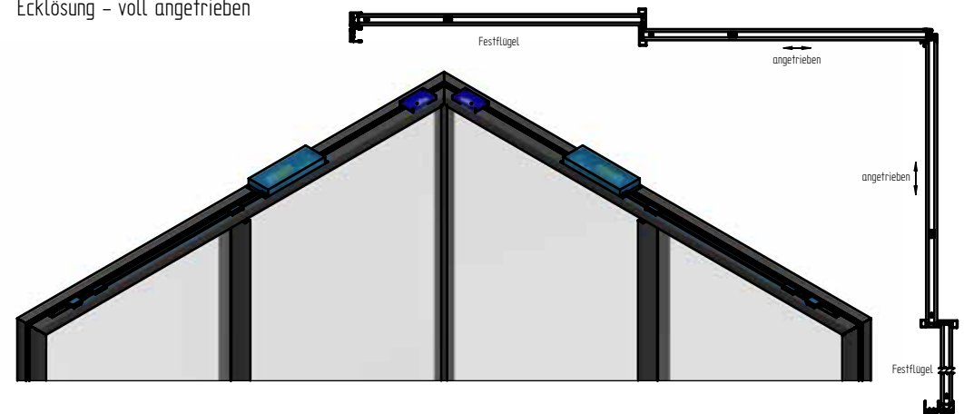
Ecklösung - voll angetrieben
